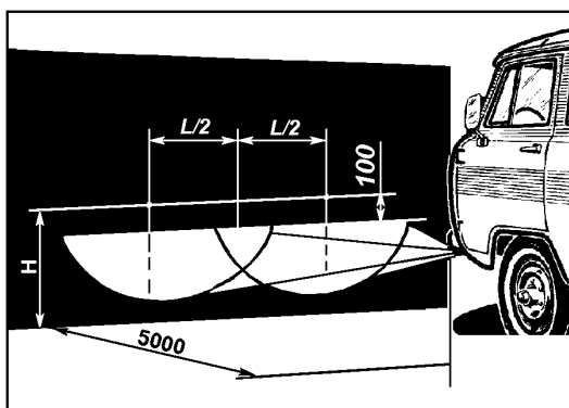
Рис. 9.43. Разметка экрана для регулировки противотуманных фар: H -расстояние от центра фар до уровня земли; L -расстояние между центрами противотуманных фар
