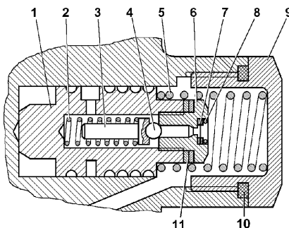
Рис. 9.29. Расходный и предохранительный клапаны насоса: 1 -золотник расходного клапана; 2 -пружина предохранительного клапана; 3 -направляющая пружины предохранительного клапана; 4-шарик предохранительного клапана; 5 -пружина золотника; 6-седло предохранительного клапана; 7 -фильтр; 8 -кольцо; 9 -пробка-заглушка; 10 -прокладка уплотнительная; 11 -прокладки регулировочные
