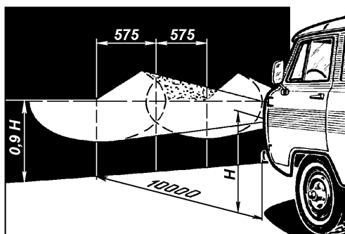
Рис. 9.42. Разметка экрана для регулировки фар: H - расстояние центра фар от уровня земли
