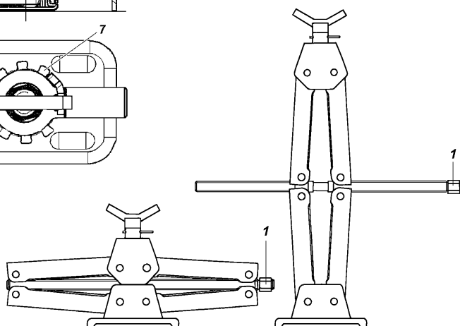
Рис. 10.2. Домкрат: 1 - шестигранный под ключ "22"
