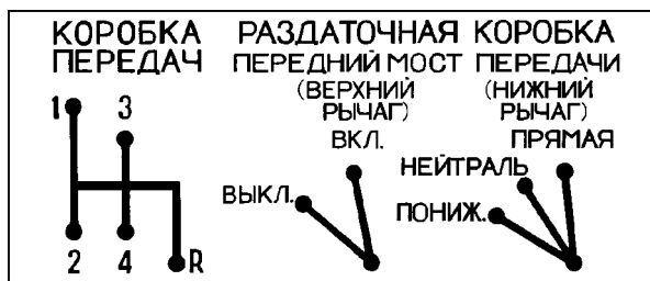
Рис. 3.4. Схема положений рычагов коробки передач и рычагов раздаточной коробки
