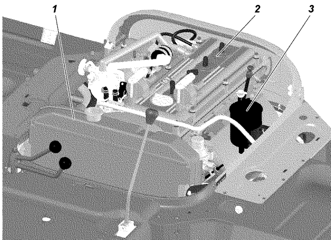
Рис. 9.28. Подкапотное пространство:
