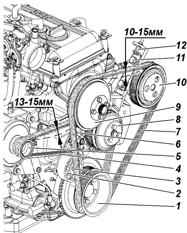
Рис. 9.5. Натяжение ремней привода агрегатов:
