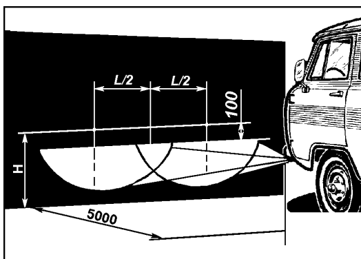
Рис. 9.42. Разметка экрана для регулировки противотуманных фар: H - расстояние от центра фар до уровня земли; L - расстояние между центрами противотуманных фар
