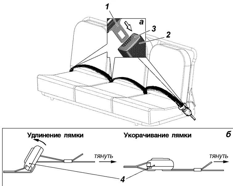
Рис. 3.6. Ремни безопасности салона автомобиля YA3-220695: 1 -язычок; 2 -замок; 3 -кнопка замка; 4 -инерционная катушка
