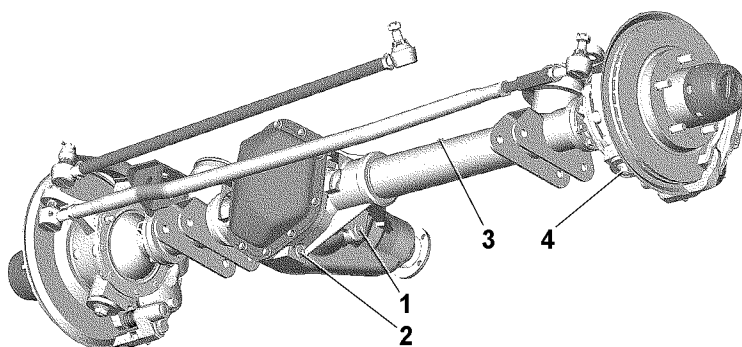
Рис. 9.18. Передний мост с неразъемным картером: 1 -пробка заливного отверстия; 2 -пробка сливного отверстия; 3 - предохранительный клапан; 4 -нижняя гайка шкворня Примечание. Возможна установка на часть автомобилей
