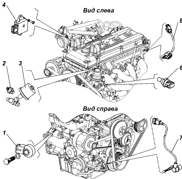
Рис. 9.8. Расположение датчиков на двигателе:
