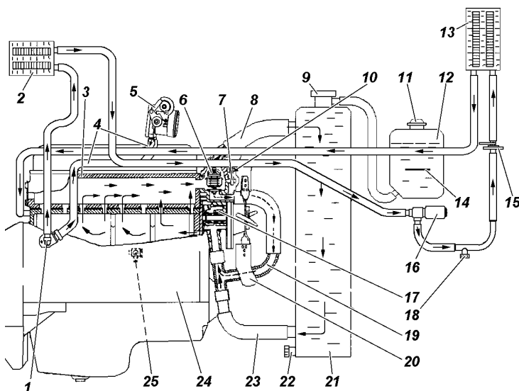
Рис. 3.8. Схема системы охлаждения двигателя и отопления кузова (ЕВРО-3): 1 -штуцер подачи охлаждающей жидкости в отопитель; 2 - радиатор отопителя салона; 3 -головка блока цилиндров; 4 -шланги подогрева дроссельного устройства; 5 -дроссельное устройство; 6 - двухклапанный термостат; 7 -датчик указателя температуры охлаждающей жидкости; 8 -подводящий шланг радиатора; 9 -заливная горловина; 10 -датчик температуры охлаждающей жидкости; 11 -пробка; 12 -расширительный бачок; 13 -радиатор отопителя кабины; 14 -отметка "min"; 15 -краник системы отопления; 16+ -электродвигатель с насосом; 17 -насос с крыльчаткой; 18 -сливная пробка (или кран) отопителя; 19 -соединительный патрубков; 20 -вентилятор; 21 -радиатор; 22 -сливная пробка радиатора; 23 -отводящий шланг радиатора; 24 -блок цилиндров; 25 -сливной кран (или пробка) блока цилиндров (находится с левой стороны двигателя)
