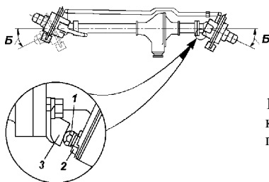
Рис. 9.19. Регулировка угла поворота колес:
