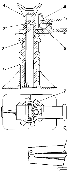
Рис. 10.1. Домкрат: 1 - корпус; 2 - наружный винт; 3 - внутренний винт; 4 - головка; 5 - "собачка"; 6 - ручка; 7 - храповик
