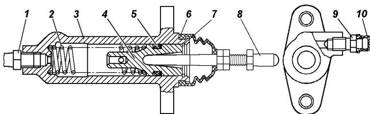
Рис. 9.12. Цилиндр выключения сцепления:
