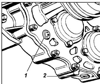
Рис. 9.15. Пробки раздаточной коробки: 1 -пробка заливного отверстия; 2 -пробка сливного отверстия
