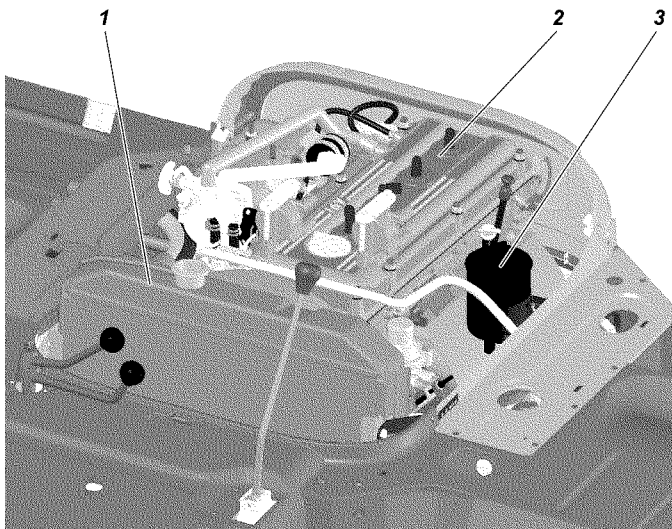
Рис. 9.28. Подкапотное пространство:
