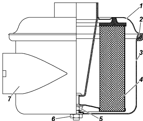
Рис. 9.13. Воздушный фильтр:
