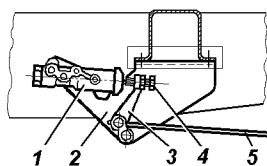
Рис. 9.35. Привод регулятора давления: 1 -регулятор давления; 2 -кронштейн (основание); 3 -рычаг привода; 4 -регулирующий болт; 5 -упругий рычаг; 6 -стойка рычага
