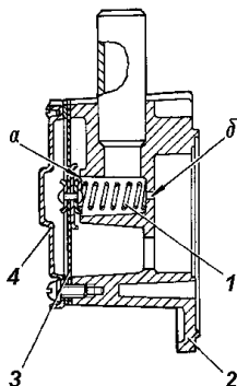
Рис. 9.6. Регулятор разрежения:
