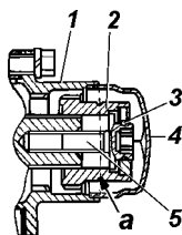
Рис. 9.21. Муфта отключения передних колес (вариантное исполнение):
