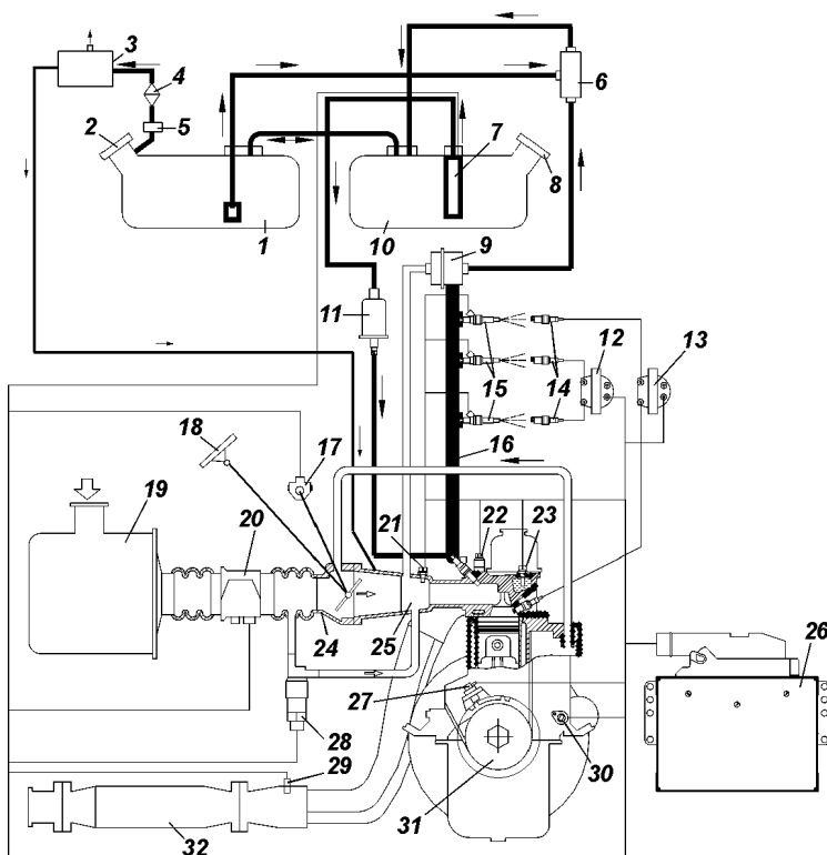
Рис. 9.9. Принципиальная схема системы питания и управления двигателем с впрыском бензина (экологический класс 2):
