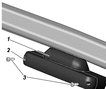
Рис. 9.49. Фонарь дополнительного сигнала торможения (UAZ PATRIOT): 1 -накладка фонаря; 2 -крышка фонаря; 3 -винты
