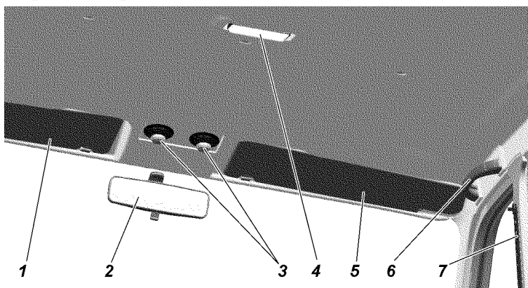
Рис. 3.17. Плафоны освещения, внутреннее зеркало заднего вида, противосолнечные козырьки и поручень:
