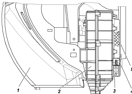
Рис. 3.16. Вентилятор:
