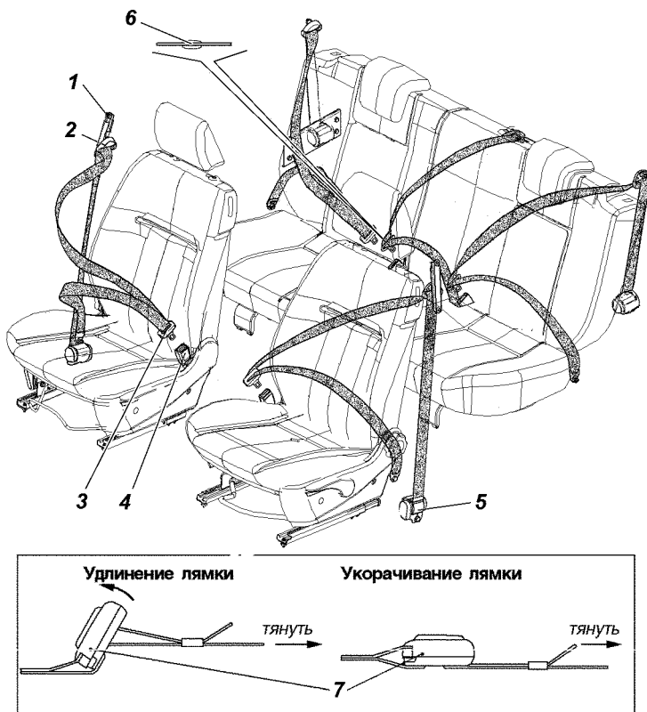
Рис. 3.28. Ремни безопасности:
