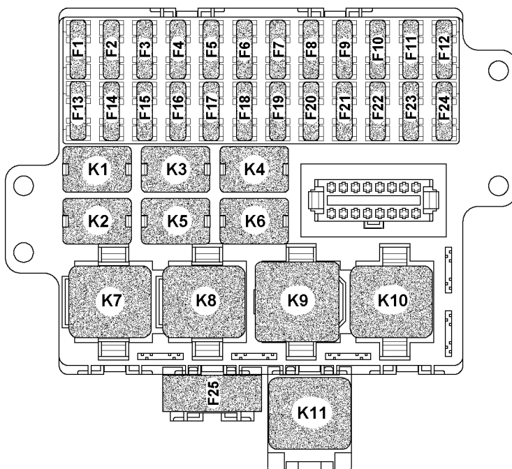
Рис. 9.39. Блок реле и предохранителей в салоне автомобиля: К1 -реле включения противотуманных фар; К2 -реле включения обогрева стекла двери задка и зеркал; К3 -реле включения дальнего света фар; К4 -реле включения ближнего света фар; К5 -реле дополнительного электронасоса отопителя (для автомобиля с двигателем ЗМЗ-40905); К6 -реле компрессора кондиционера; К7 -прерыватель указателей поворота и аварийной сигнализации; К8 -прерыватель стеклоочистителя с программируемой паузой; К9 -дополнительное (разгрузочное) реле; К10 -реле обогрева ветрового стекла (разгрузочное) или реле переключения топливных баков (для автомобилей с РК "УАЗ"); К11 -реле времени обогрева ветрового стекла; F1-F25 -плавкие предохранители (см. таблицу)
