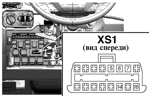
Рис. 9.10 Диагностический разъем (XS1): 5 -масса; 6, 14 -Сен-линия; 7 -К-линия; 16 -+12В
