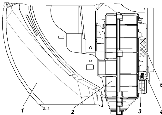
Рис. 3.15. Вентилятор:
