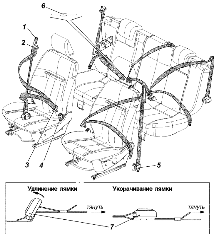
Рис. 3.25. Ремни безопасности:
