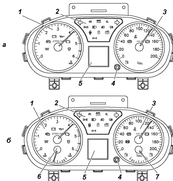
Рис. 3.5. Комбинация приборов (наименование позиций см. в тексте):
