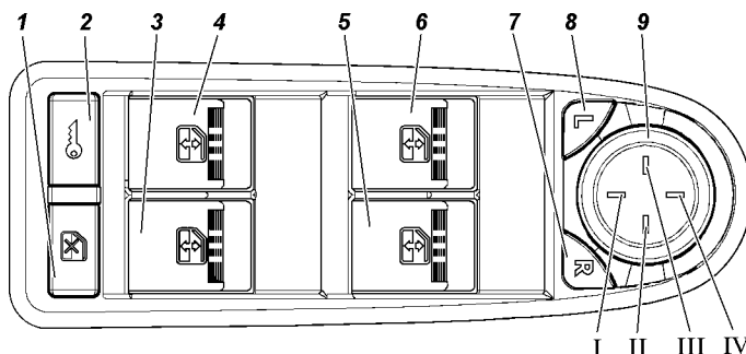
Рис. 3.9. Модуль переключателей двери водителя с мультиплексным управлением:
