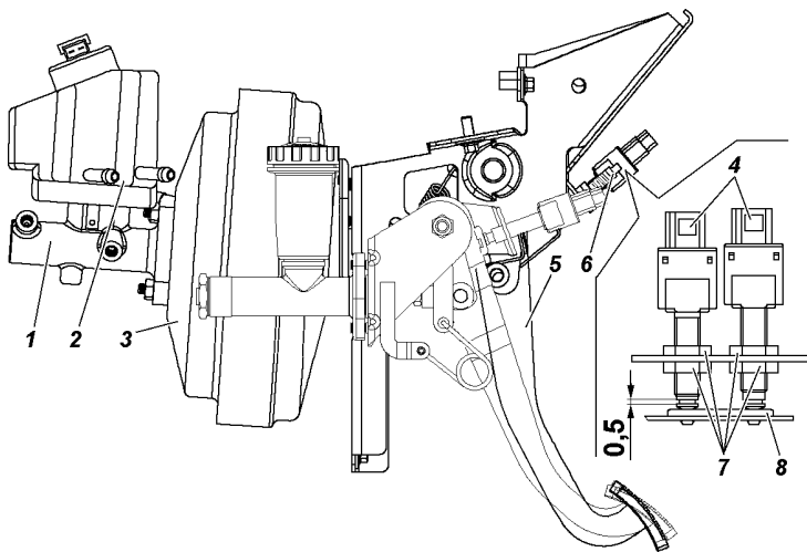
Рис. 9.36. Привод главного тормозного цилиндра: 1 -картер главного тормозного цилиндра; 2 -бачок; 3 -вакуумный усилитель; 4 -выключатели сигнала торможения; 5 -педаль тормоза; 6 - гайки; 7 -буфер
