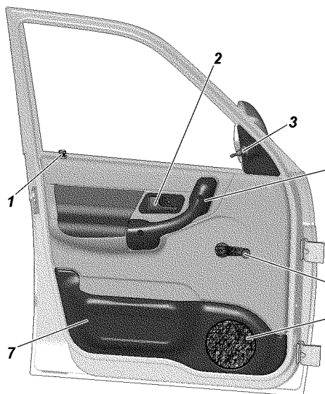
Рис. 3.18. Передняя дверь:
