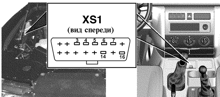
Рис. 9.21. Диагностический разъем (XS1): 3 -автоматический режим для тестера EASY; 4, 5 -масса; 6, 14 -Сиг- линия; 7 -К-линия; 16 -+12В
