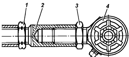
Рис. 9.28. Тяга рулевой трапеции:
