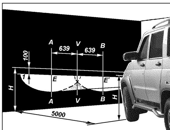
Рис. 9.44. Разметка экрана для регулировки противотуманных фар: H - расстояние центра фар от уровня земли; V-V - проекция продольной оси автомобиля; A-A, B-B - оси центров фар
