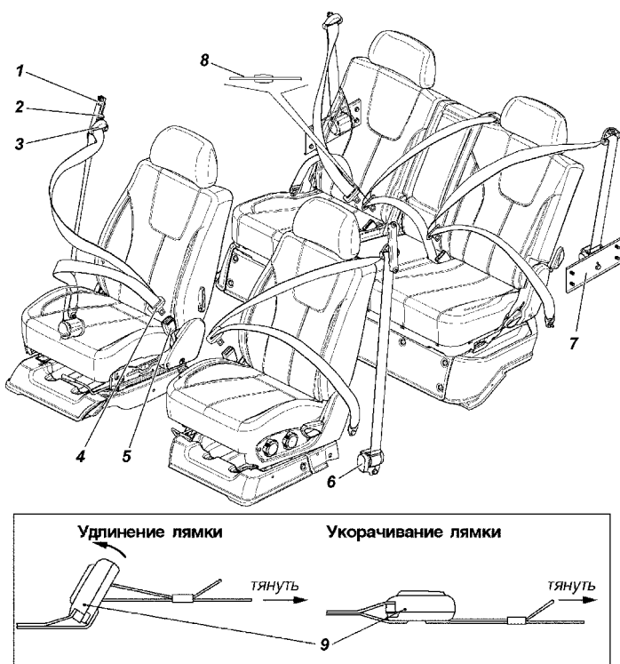
Рис. 3.25. Ремни безопасности:
