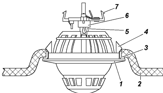
Рис. 9.51. Плафоны индивидуального освещения: 1 -корпус плафона; 2 -обивка крыши; 3 -установочное кольцо; 4 - защелка плафона; 5 -лампа; 6 -патрон; 7 -защелка патрона
