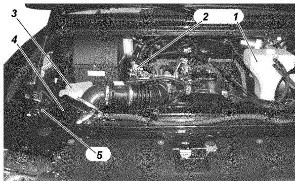
Рис. 3.26. Подкапотное пространство (фрагмент):
