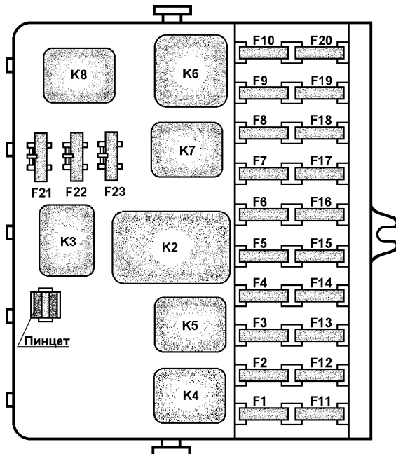
Рис. 9.38. Монтажный блок:
