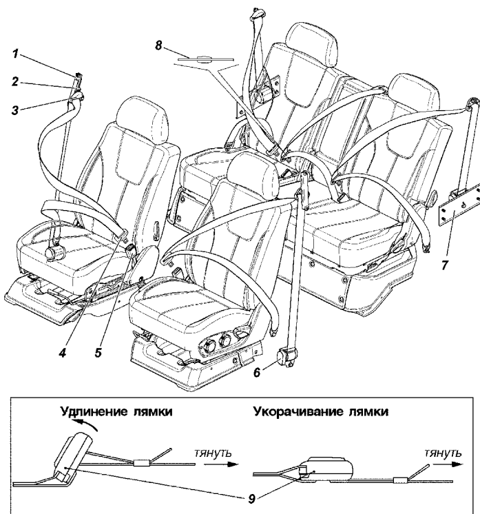
Рис. 3.27. Ремни безопасности:
