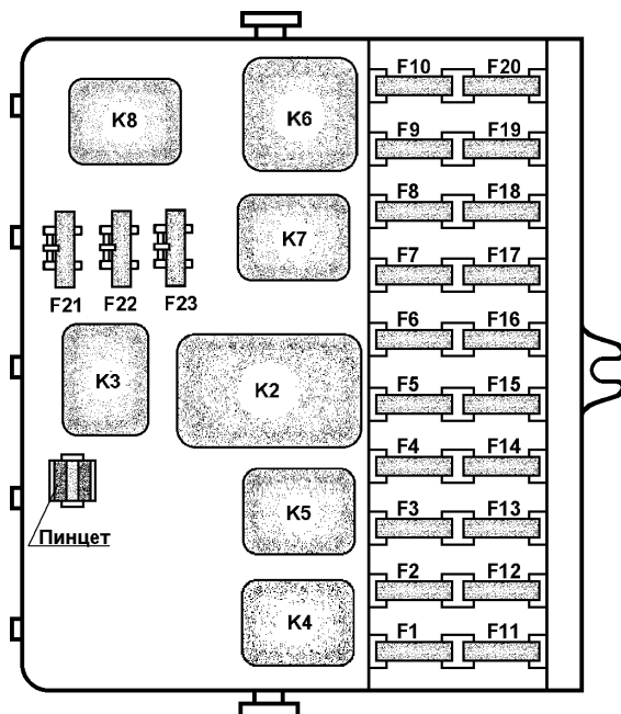
Рис. 9.37. Монтажный блок:
