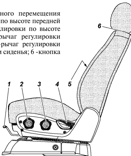
Рис. 3.22. Переднее сиденье:
