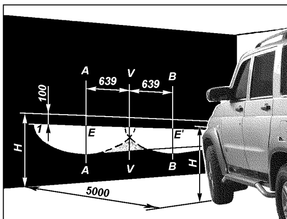
Рис. 9.43. Разметка экрана для регулировки противотуманных фар: H - расстояние центра фар от уровня земли; V-V - проекция продольной оси автомобиля; A-A, B-B - оси центров фар
