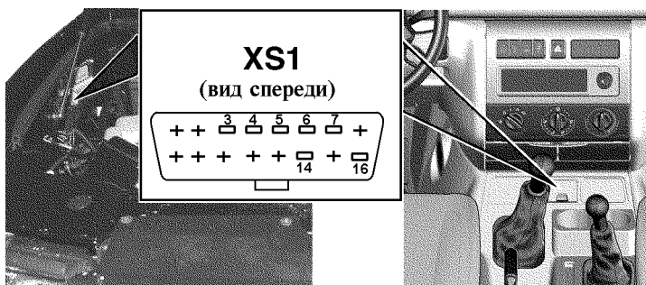
Рис. 9.21. Диагностический разъем (XS1): 3 -автоматический режим для тестера EASY; 4, 5 -масса; 6, 14 -Can- линия; 7 -К-линия; 16 -+12В
