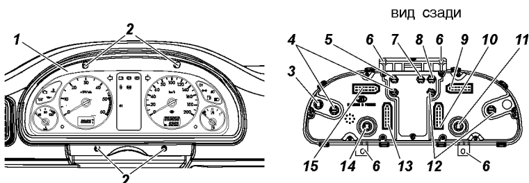
Рис. 9.52. Комбинация приборов:
