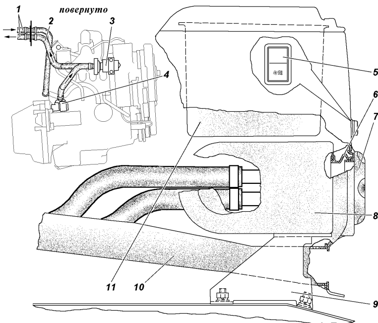
Рис. 3.11. Дополнительный отопитель:
