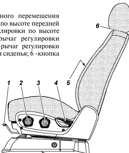
Рис. 3.17. Переднее сиденье:
