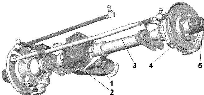
Рис. 9.17. Передний мост:
