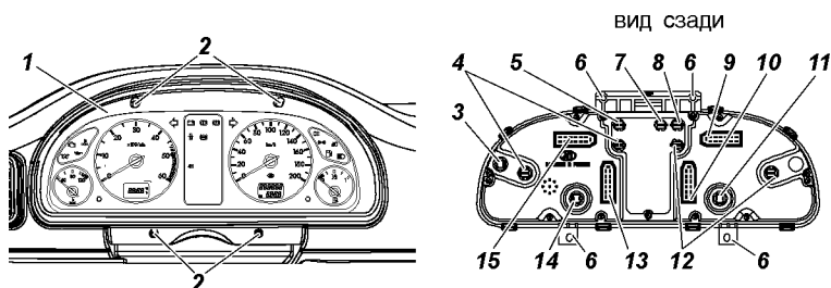
Рис. 9.44. Комбинация приборов:
