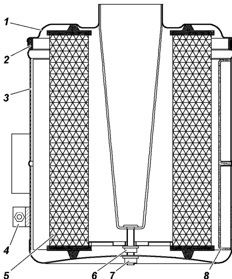
Рис. 9.12. Воздушный фильтр:
