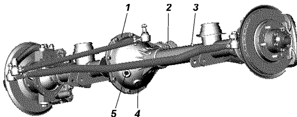
Рис. 9.27. Передний мост:
