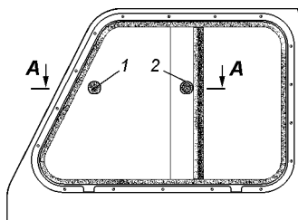
Рис. 3.6. Надставка двери:
