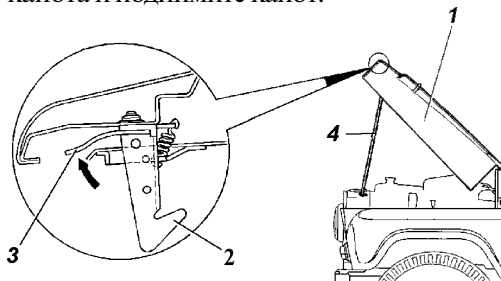
Рис. 3.10. Капот: 1 -капот; 2 -предохранитель открывания капота; 3 -рычаг предохранителя; 4 -упор капота.
