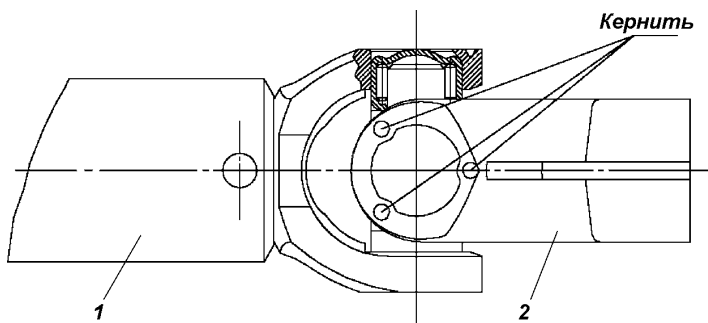
Рис. 9.36. Раскерновка подшипников: 1 -вал карданный; 2 -вилка карданного вала.
