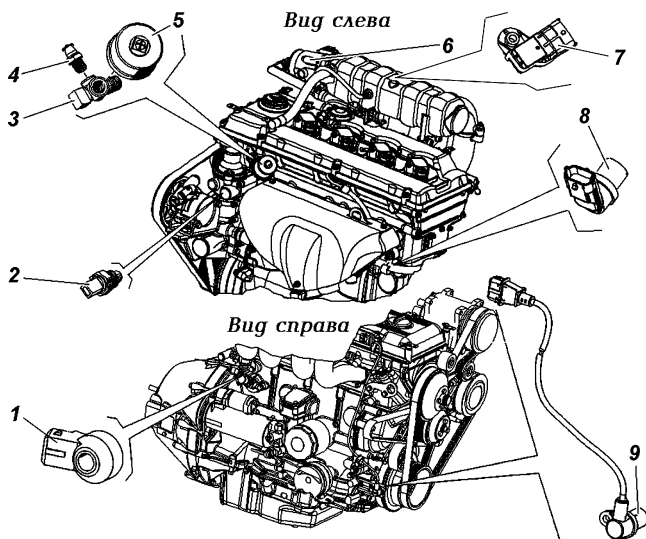
Рис. 9.7. Расположение датчиков на двигателе:
