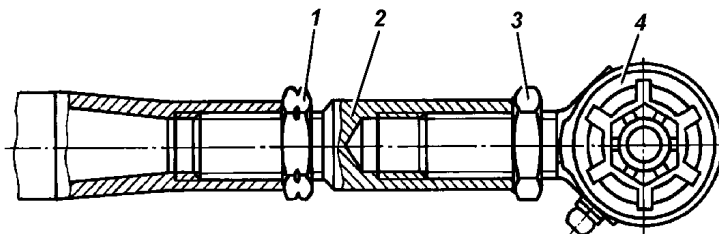
Рис. 9.33. Тяга рулевой трапеции:
