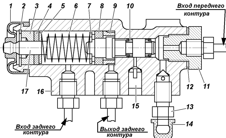
Рис. 9.41. Регулятор давления:
