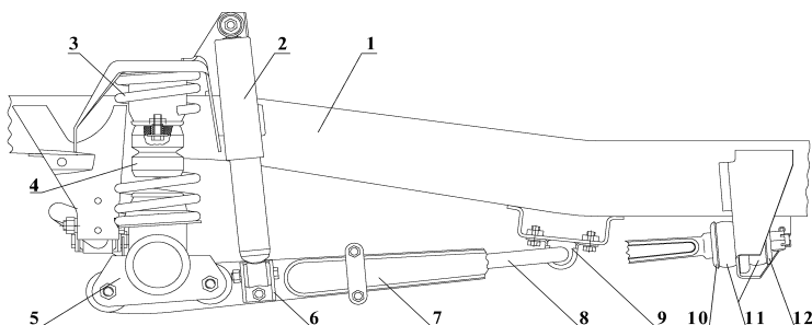
Рис. 9.30. Передняя зависимая пружинная подвеска:
