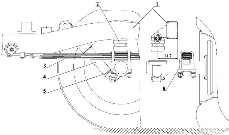
Рис. 9.49. Подвеска задняя:
