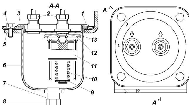
Рис. 9.7. Топливный фильтр-отстойник:
