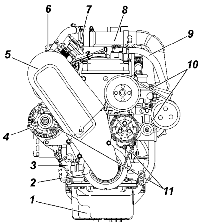
Рис. 9.31. Вид спереди (вентилятор и муфта привода вентилятора условно сняты):
