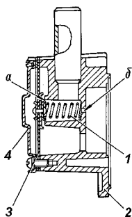
Рис. 9.6. Регулятор разрежения:
