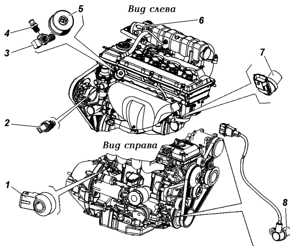
Рис. 9.25. Расположение датчиков на двигателе 3М3-409 (Экологический класс 3):
