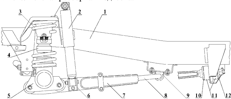
Рис. 9.48. Передняя зависимая пружинная подвеска:
