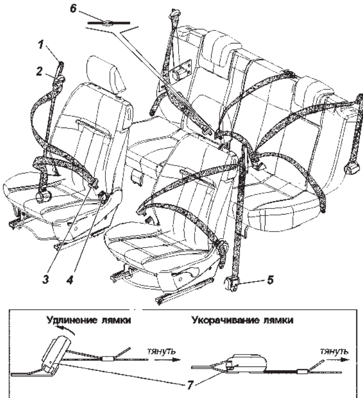
Рис. 3.39. Ремни безопасности:
