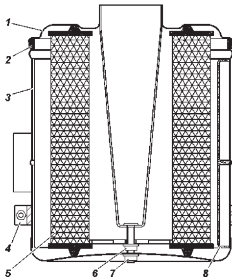
Рис. 9.10. Воздушный фильтр:
