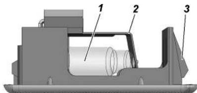
Рис. 9.44. Плафон подсветки вещевого ящика: 1 -лампа; 2 -держатель лампы; 3 -фиксаторы
