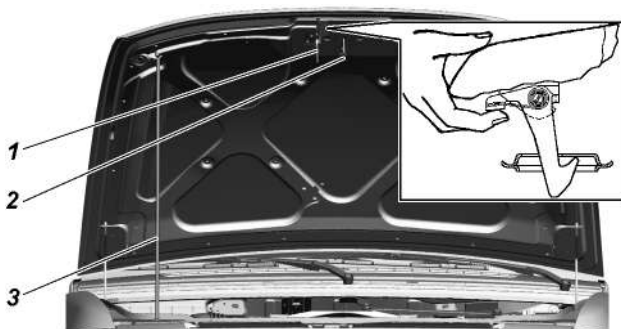
Рис. 3.44. Капот: 1 -запорный крючок; 2 -держатель; 3 -упор
