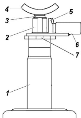
Рис. 10.1. Домкрат:
