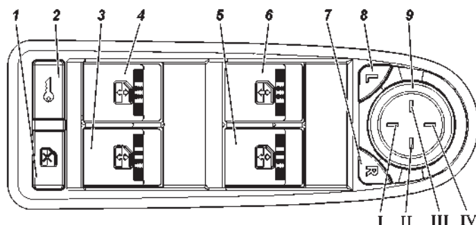
Рис. 3.15. Модуль переключателей двери водителя с мультиплексным управлением: 1 -выключатель блокировки стеклоподъемников на дверях пассажиров; 2 -выключатель центральной блокировки дверей; 3 -выключатель управления стеклоподъемником задней правой двери; 4 -выключатель управления стеклоподъемником задней левой двери; 5 -выключатель управления стеклоподъемником передней правой двери; 6 -выключатель управления стеклоподъемником двери водителя; 7 -выключатель выбора правого зеркала; 8 -выключатель выбора левого зеркала; 9 -переключатель управления положением наружных зеркал заднего вида: I -зеркало вниз; II -зеркало вправо; III -зеркало влево; IV -зеркало вверх
