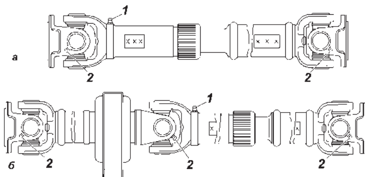
Рис. 9.14. Карданный вал:
