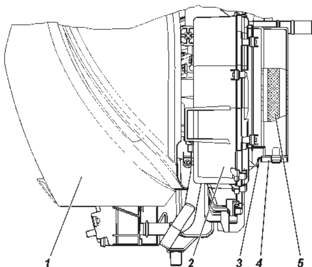
Рис. 3.28. Вентилятор:
