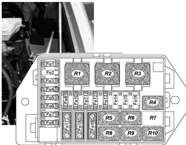
Рис. 9.32. Блок реле и предохранителей под капотом автомобиля(без крышки): R1-R10 -реле; Fe1-Fe19 -плавкие предохранители (см. таблицу 9.1)
