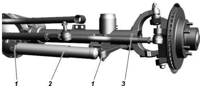
Рис. 9.18. Установка демфера (для УАЗ ПАТРИОТ): 1 -резинометаллические шарниры; 2 -демфер; 3 -передний мост
