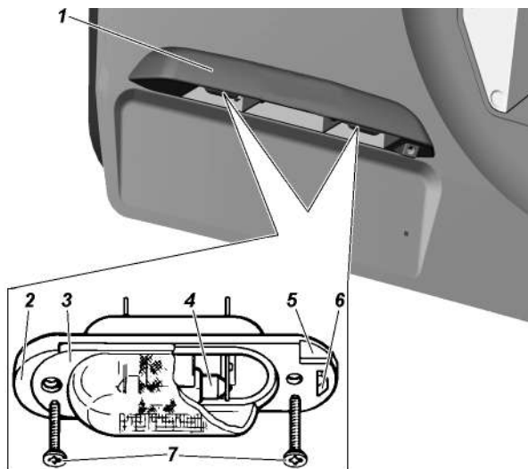
Рис. 9.40. Фонари освещения номерного знака: 1 - накладка фонарей освещения номерного знака; 2 - корпус фонаря; 3 -рассеиватель фонаря; 4 -лампа; 5 -паз; 6 -защелка 7 -винты
