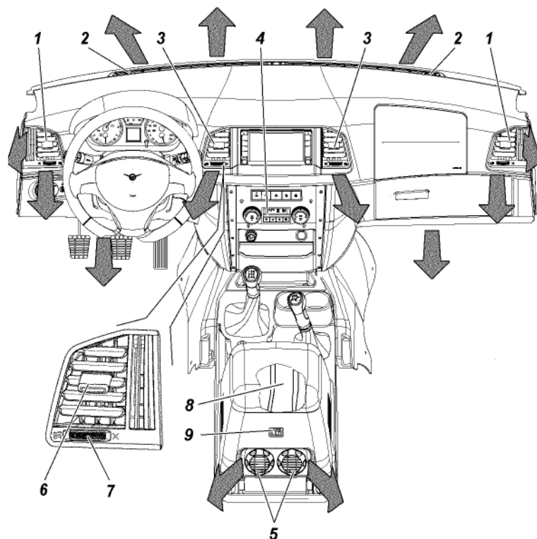
Рис. 3.25. Органы управления системой вентиляции и отопления салона(наименование позиций см. в тексте)
