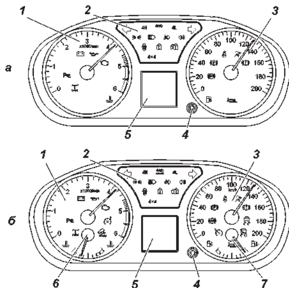
Рис. 3.4. Комбинация приборов (наименование позиций см. в тексте): а - двух стрелочная; б - четырех стрелочная
