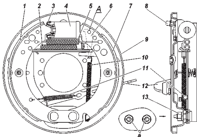
Рис. 9.23. Тормоз заднего колеса под колесный стояночный тормоз (Вариантное исп. 1): а -метки на опорных пальцах; 1, 7 -тормозные колодки с накладкой; 2 -пружина разжимного звена; 3 -защитный колпак; 4 -колесный тормозной цилиндр; 5 -пружина стяжная колодок; 6 -клин регулировочный; 8 -перепускной клапан; 9 -щит; 10 -пружина регулировочного клина; 11 -пружина приводного рычага; 12 -блок промежуточного рычага; 13 - опорные пальцы
