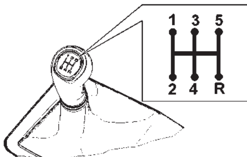
Рис. 3.22. Схема положений рычага коробки переключения передач
