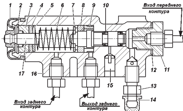
Рис. 9.25. Регулятор давления:
