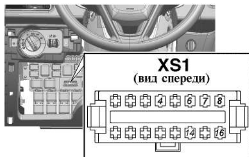
Рис. 9.11. Диагностический разъем (XS1): 4 -масса; 6, 14 -Сap-линия; 7 -K-линия; 16 -+12B; 8 -диагностика ПК «Divgi TTS» обслуживания.
