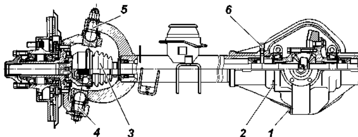
Рис. 9.15. Передний мост с поворотными кулаками открытого типа:
