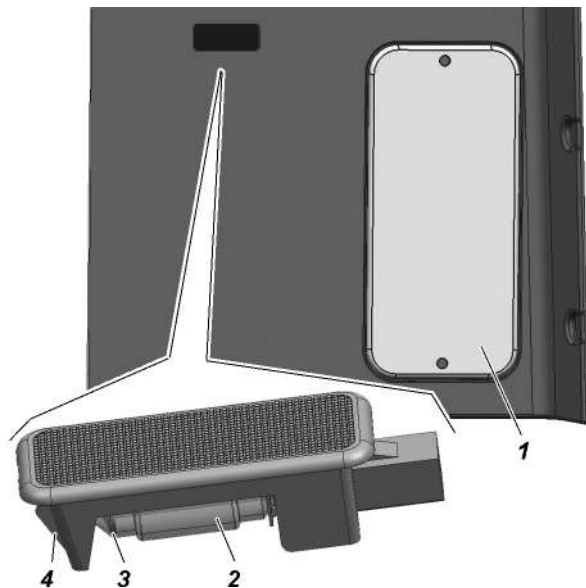
Рис. 9.45. Плафон освещения багажника: 1 -крышка; 2 -лампа; 3 -держатель лампы; 4 -фиксаторы
