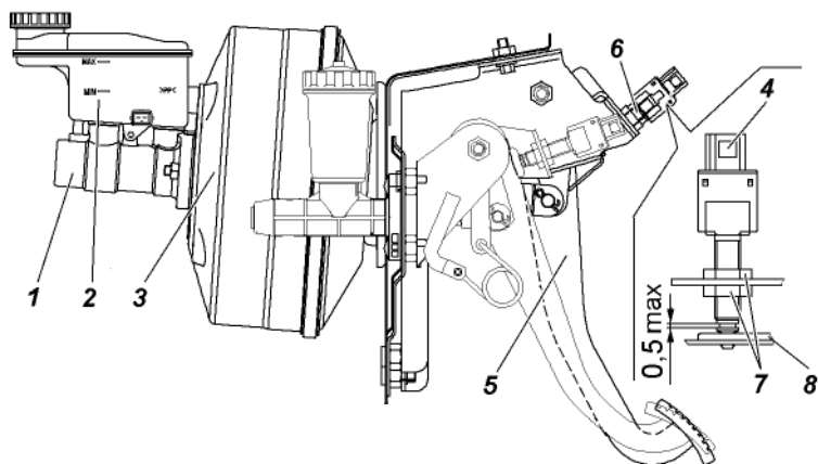
Рис. 9.27. Привод главного тормозного цилиндра: 1 -картер главного тормозного цилиндра; 2 -бачок; 3 -вакуумный усилитель; 4 -выключатели сигнала торможения; 5 -педаль тормоза; 6 -винт регулировочный; 7 -гайки; 8 -буфер
