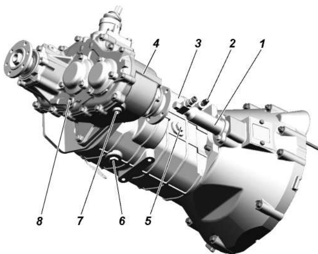
Рис. 9.13. Пятиступенчатая коробка передач «BAIC», раздаточная коробка ООО «УАЗ» и рабочий цилиндр выключения сцепления:
