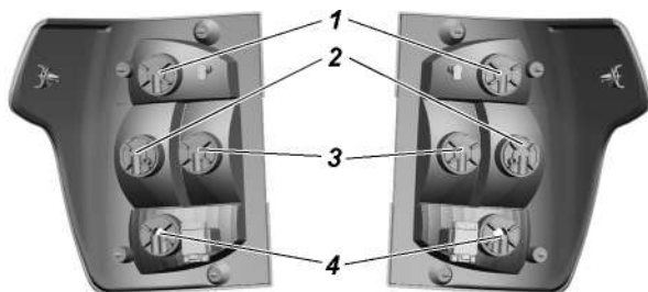
Рис. 9.39. Задние фонари: 1 -патрон лампы сигнала торможения; 2 -патрон лампы указателей поворота; 3 -патрон лампы света заднего хода; 4 -патрон лампы противотуманного и габаритного огня
