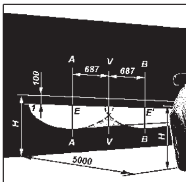
Рис. 9.36. Разметка экрана для регулировки противотуманных фар: H - расстояние центра фар от уровня земли; V-V - проекция продольной оси автомобиля; A-A, B-B - оси центров фар
