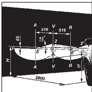
Рис. 9.33. Разметка экрана для регулировки фар: Н -расстояние центра фар от уровня земли; V-V -проекция продольной оси автомобиля; А-А, В-В - оси центров фар
