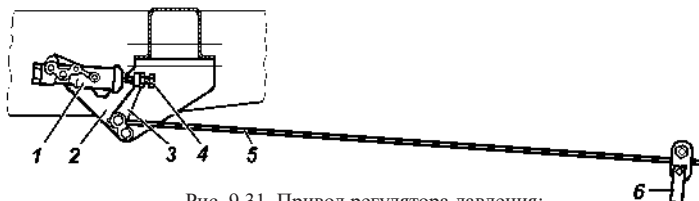
Рис. 9.31. Привод регулятора давления:
