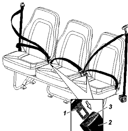
Рис. 3.11. Ремни безопасности салона автомобиля УАЗ-390995, УАЗ-390945: 1 -язычок; 2 -замок; 3 -кнопка замка
