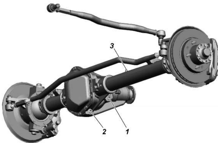
Рис. 9.17. Передний мост с неразъемным картером: 1 -пробка заливного отверстия; 2-пробка сливного отверстия; 3-предохранительный клапан
