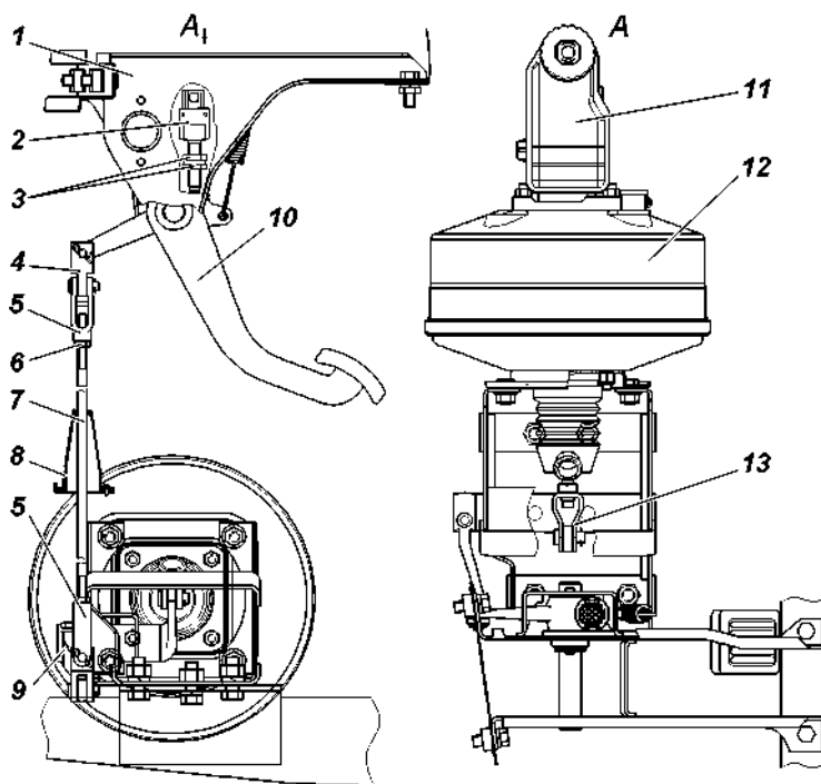
Рис. 9.32. Привод главного тормозного цилиндра:
