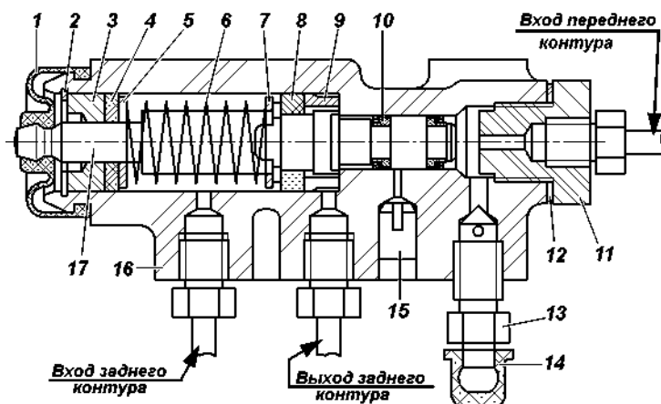
Рис. 9.30. Регулятор давления:
