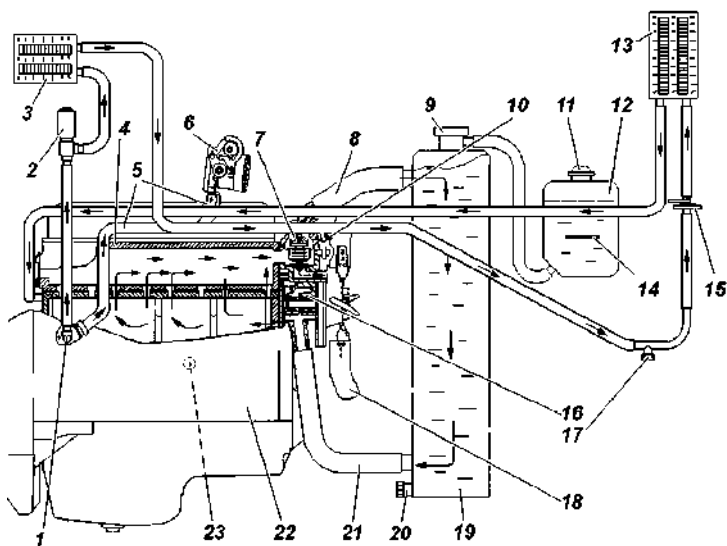
Рис. 3.12. Схема системы охлаждения двигателя и отопления кузова:
