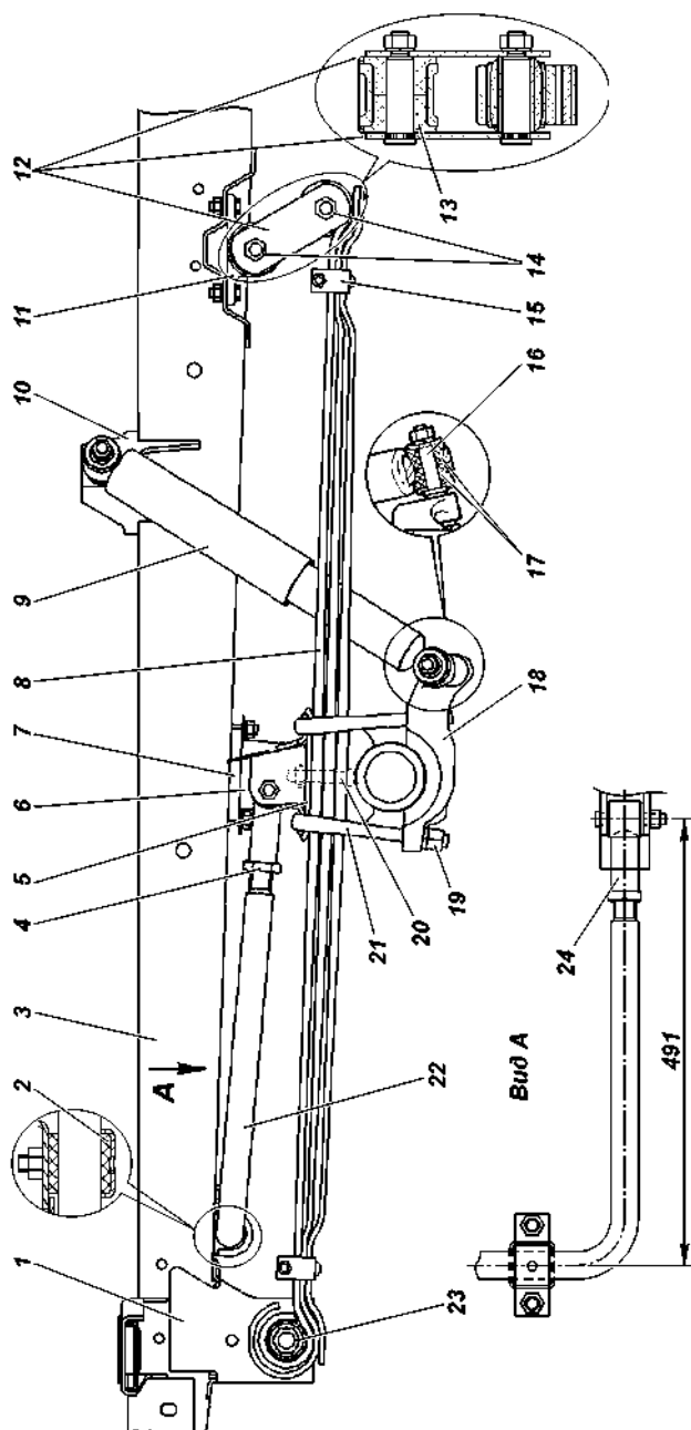
Рис. 9.21. Передняя подвеска автомобилей:
