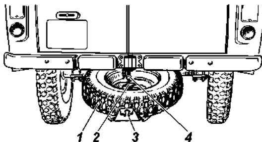
Рис. 9.23. Крепление запасного колеса:
