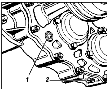
Рис. 9.14. Пробки раздаточной коробки: 1 -пробка заливного отверстия; 2 -пробка сливного отверстия
