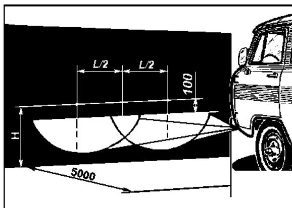
Рис. 9.40. Разметка экрана для регулировки противотуманных фар:
