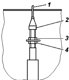
Рис. 9.8. Регулировка привода педали дроссельной заслонки : 1 -трос; 2 -оболочка троса с регулировочным наконечником; 3, 4 -гайки
