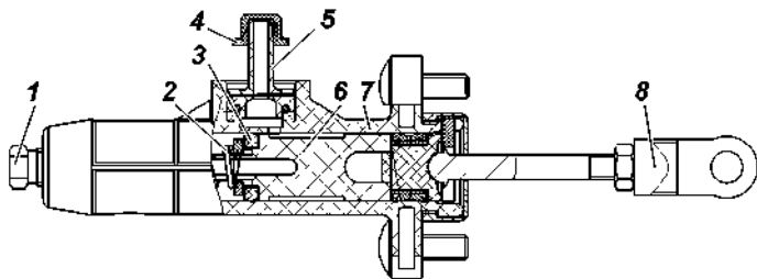
Рис. 9.11. Цилиндр выключения сцепления:
