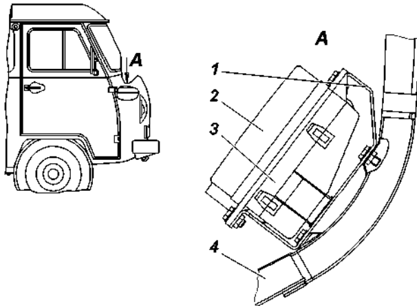
Рис. 9.35. Расположение блока реле и предохранителей: 1 -кронштейн; 2 -крышка блока реле и предохранителей; 3 -блок реле и предохранителей; 4 -рейка панели передка
