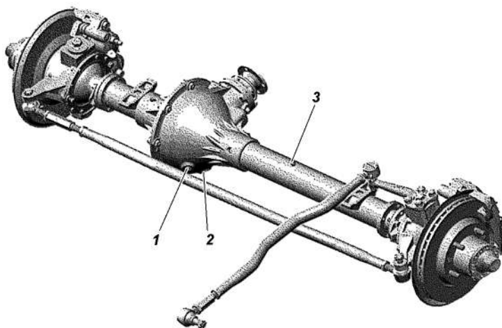
Рис. 9.16. Передний мост с разъемным в вертикальной плоскости картером: 1 -пробка заливного отверстия; 2 -сливная пробка; 3 -предохранительный клапан
