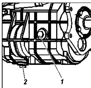
Рис. 9.13. Пробки коробки передач: 1 -пробка заливного отверстия; 2 -пробка сливного отверстия
