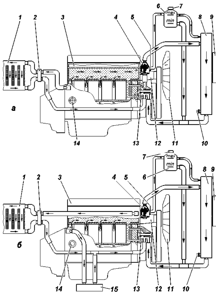
Рис. 9.5. Схема системы охлаждения двигателя и отопления:
