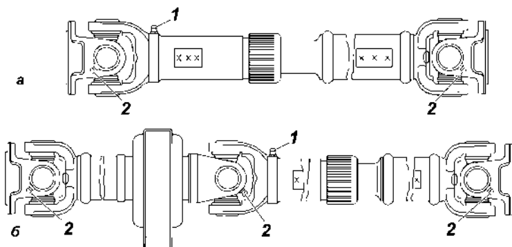
Рис. 9.16. Карданный вал:
