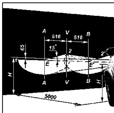
Рис. 9.38. Разметка экрана для регулировки фар: Н -расстояние центра фар от уровня земли; V-V -проекция продольной оси автомобиля; А-А, В-В - оси центров фар
