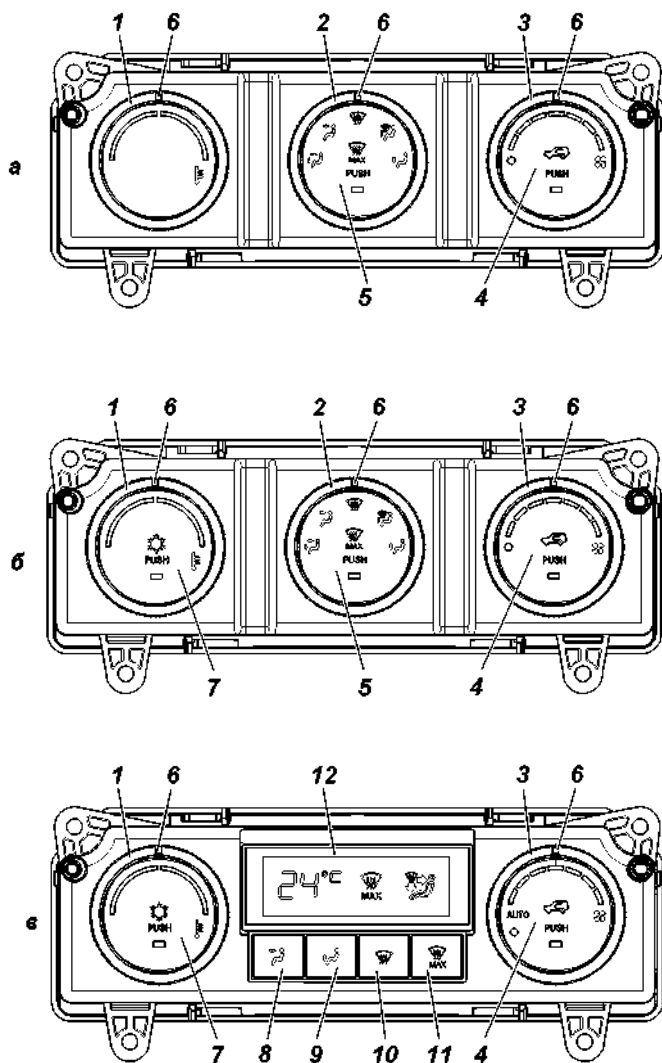
Рис. 3.35. Пульт управления отопителем:
