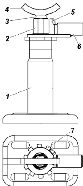
Рис. 10.1. Домкрат:
