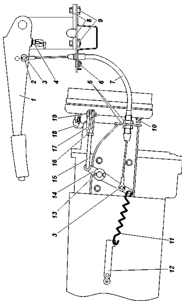
Рис. 9.33. Привод стояночного тормоза трансмиссионный:
