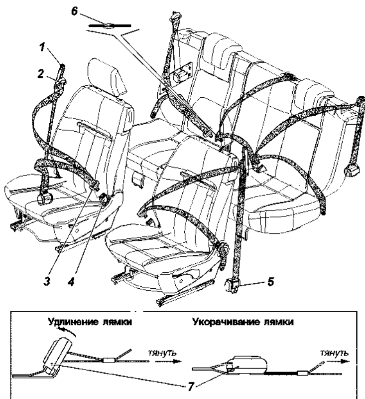
Рис. 3.49. Ремни безопасности:
