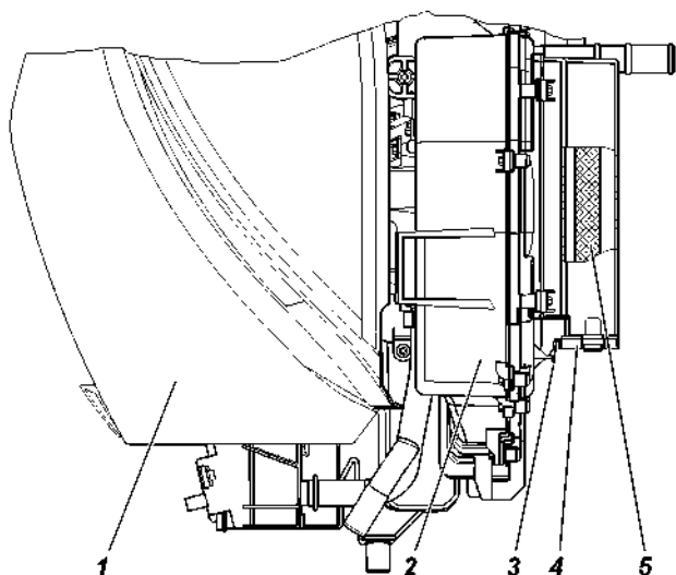
Рис. 3.38. Вентилятор:
