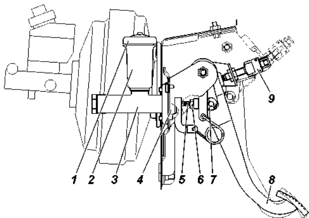
Рис. 9.12. Привод главного цилиндра выключения сцепления:
