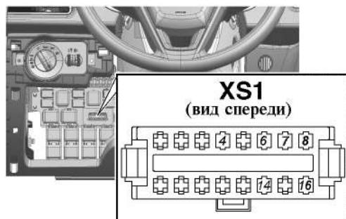
Рис. 9.11. Диагностический разъем (XS1): 4 -масса; 6, 14 -Сap-линия; 7 -К-линия; 16 -+12В; 8 -диагностика ПК «Divgi TTS»
