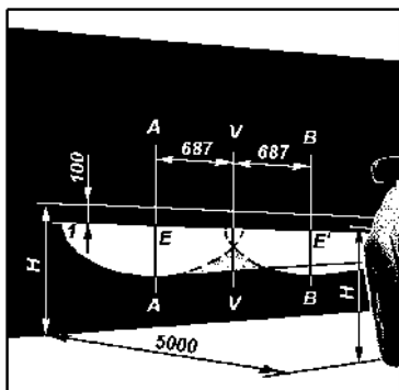
Рис. 9.41. Разметка экрана для регулировки противотуманных фар: H - расстояние центра фар от уровня земли; A-A, B-B - проекция продольной оси автомобиля; V-V - проекция продольной оси фар
