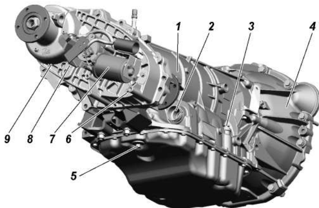
Рис. 3.28. Автоматическая коробка передач «Punch», раздаточная коробка «Divgi TTS»: 1 -автоматическая коробка передач (АКП); 2 -патрубок разъема электрооборудования; 3 -пробка наливного патрубка; 4 -картер гидротрансформатора; 5 -пробка сливного отверстия картера АКП; 6 -пробка сливного отверстия картера раздаточной коробки; 7 -электропривод; 8 -пробка заливного отверстия картера раздаточной коробки; 9 -раздаточная коробка
