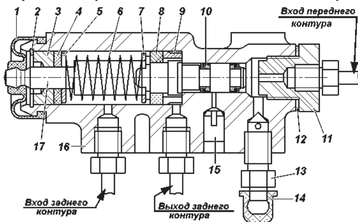
Рис. 9.32. Регулятор давления:
