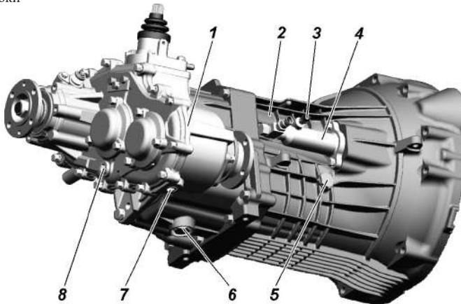
Рис. 9.19. Рабочий цилиндр выключения сцепления, пятиступенчатая коробка передач «Dumos» и раздаточная коробка: 1 -раздаточная коробка; 2 -коробка передач; 3 -клапан перепускной; 4 -цилиндр выключения сцепления; 5 -пробка заливного отверстия картера коробки передач; 6 -пробка сливного отверстия картера коробки передач; 7 -пробка сливного отверстия картера раздаточной коробки; 8 -пробка заливного отверстия картера раздаточной коробки
