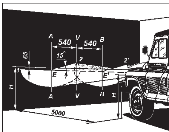
Рис. 9.37. Разметка экрана для регулировки фар: Н - расстояние центра фар от уровня земли; V-V - проекция продольной оси автомобиля; А-А, В-В - оси центров фар
