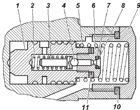
Рис. 9.28. Расходный и предохранительный клапаны насоса: 1 -золотник расходного клапана; 2 -пружина предохранительного клапана; 3 -направляющая пружины предохранительного клапана; 4 -шарик предохранительного клапана; 5 -пружина золотника; 6-седло предохранительного клапана; 7 -фильтр; 8 -кольцо; 9 -пробка-заглушка; 10 -прокладка уплотнительная; 11 -прокладки регулировочные
