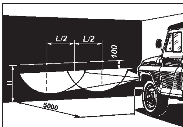
Рис. 9.38. Разметка экрана для регулировки противотуманных фар: Н - расстояние от центра фар до уровня земли; L - расстояние между центрами противотуманных фар
