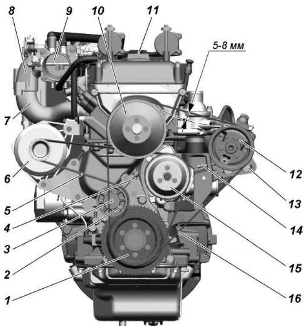
Рис. 9.13. Натяжение ремней привода агрегатов:
