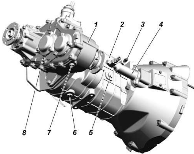
Рис. 9.18. Пятиступенчатая коробка передач «ВАИС» и раздаточная коробка: 1 -раздаточная коробка; 2 -коробка передач; 3 -клапан перепускной; 4 -цилиндр выключения сцепления; 5 -пробка заливного отверстия картера коробки передач; 6 -пробка сливного отверстия картера коробки передач; 7 -пробка сливного отверстия картера раздаточной коробки; 8 -пробка заливного отверстия картера раздаточной коробки
