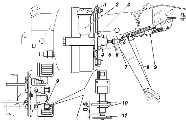
Рис. 9.17. Привод главного цилиндра выключения сцепления: 1 -крышка бачка; 2 -корпус бачка; 3 -корпус главного цилиндра; 4 -колпак защитный; 5 -толкатель; 6 -гайка; 7 -муфта толкателя; 8 -педаль выключения сцепления; 9 -выключатель педали сцепления; 10 -гайки; 11 -буфер
