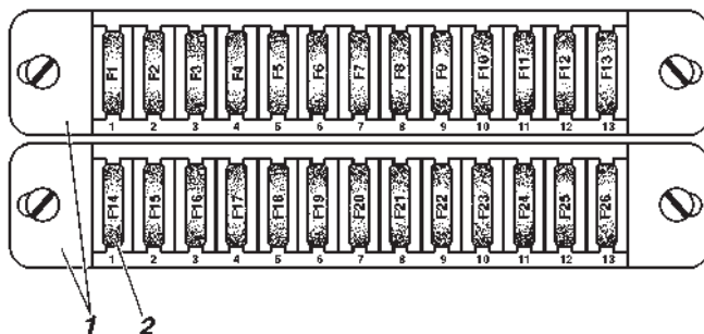
Рис. 9.39. Блок плавких предохранителей:
