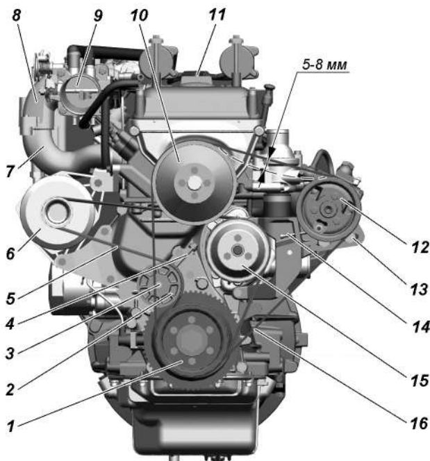
Рис. 9.13. Натяжение ремней привода агрегатов: 1 -шкив-демпфер коленчатого вала; 2 -натяжной ролик; 3 -болт крепления натяжного ролика; 4 -регулирующий болт; 5 -ремень привода водяного насоса и генератора; 6 -генератор; 7 -впускная труба; 8 -резонатор; 9 -дрессельный узел с датчиком положения дроссельной заслонки; 10 -шкив вентилятора; 11 -крышка маслоналивного патрубкa; 12 -шкив насоса ГУР; 13 -болт крепления насоса гидроусилителя рулевого управления; 14 -натяжной болт; 15 -шкив водяного насоса; 16 -ремень привода вентилятора и насоса ГУР
