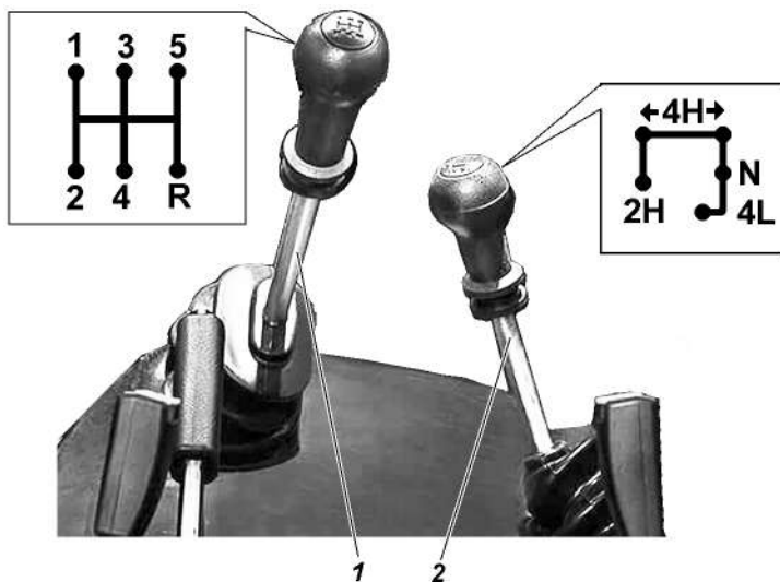
Рис. 3.5. Схема положения рычагов трансмиссии: 1 -рычаг коробки переключения передач; 2 -рычаг раздаточной коробки
