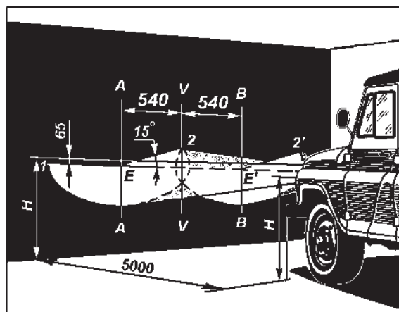
Рис. 9.37. Разметка экрана для регулировки фар: H - расстояние центра фар от уровня земли; V-V - проекция продольной оси автомобиля; A-A , B-B - оси центров фар
