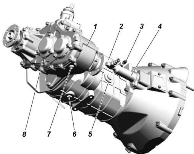
Рис. 9.18. Пятиступенчатая коробка передач «BAIC» и раздаточная коробка: 1 -раздаточная коробка; 2 -коробка передач; 3 -клапан перепускной; 4 -цилиндр выключения сцепления; 5 -пробка заливного отверстия картера коробки передач; 6 -пробка сливного отверстия картера коробки передач; 7 -пробка сливного отверстия картера раздаточной коробки; 8 -пробка заливного отверстия картера раздаточной коробки
