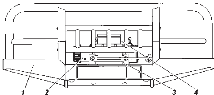
Рис. 10.2. Лебедка:
