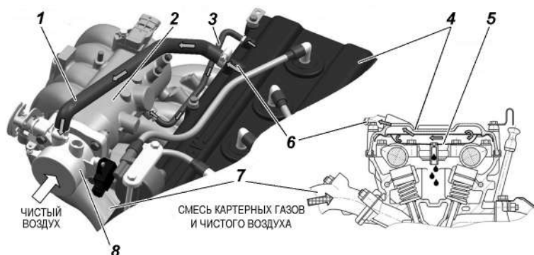
Рис. 9.12. Схема вентиляции картера двигателя:
