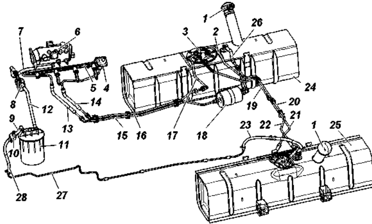
Рис. 9.15. Схема системы питания двигателя топливом: 1 -пробка топливного бака; 2,13,15,19,21 -трубки подачи топлива; 3 -топливный модуль; 4 -регулятор давления топлива; 5 -топливная рампа; 6 -дроссельное устройство; 7,9,12,23,26,28 -шланги пароотводящие; 8 -клапан продувки адсорбера; 10 -клапан бензобака; 11 -адсорбер; 14,16,17 -трубка слива топлива; 18 -фильтр тонкой очистки топлива; 20,22,27 -трубки пароотводящие; 24 -правый топливный бак; 25 -левый топливный бак
