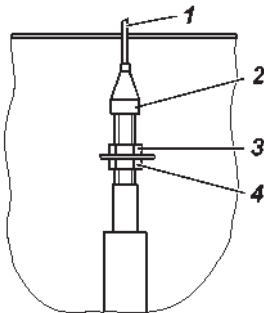
Рис. 9.16. Регулировка привода педали дроссельной заслонки : 1 -трос; 2 -оболочка троса с регулировочным наконечником; 3, 4 -гайки
