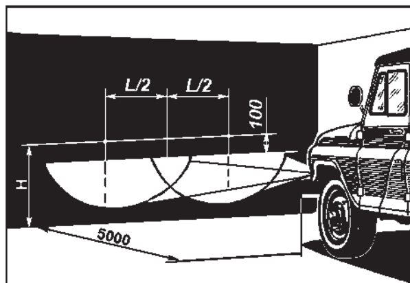
Рис. 9.38. Разметка экрана для регулировки противотуманных фар: H - расстояние от центра фар до уровня земли; L - расстояние между центрами противотуманных фар
