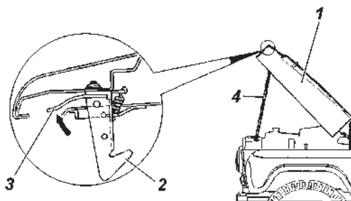
Рис. 3.14. Капот:
