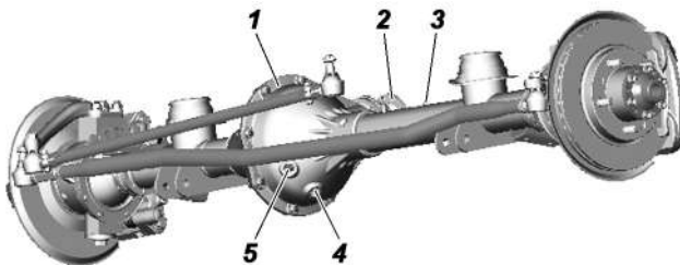
Рис. 9.22. Передний мост с вертикальным разъемом картера: 1 -картер переднего моста; 2 -фланец ведущей шестерни; 3 -клапан предохранительный; 4 -пробка сливного отверстия; 5 -пробка заливного отверстия
