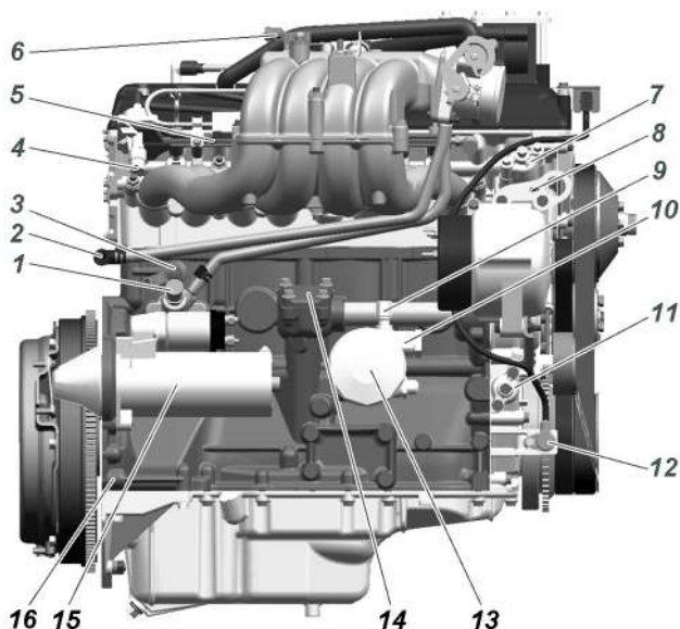
Рис. 9.11. Двигатель (вид справа):
