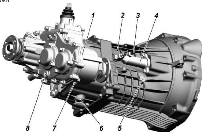
Рис. 9.19. Рабочий цилиндр выключения сцепления, пятиступенчатая коробка передач «Dymos» и раздаточная коробка: 1 -раздаточная коробка; 2 -коробка передач; 3 -клапан перепускной; 4 -цилиндр выключения сцепления; 5 -пробка заливного отверстия картера коробки передач; 6 -пробка сливного отверстия картера коробки передач; 7 -пробка сливного отверстия картера раздаточной коробки; 8 -пробка заливного отверстия картера раздаточной коробки
