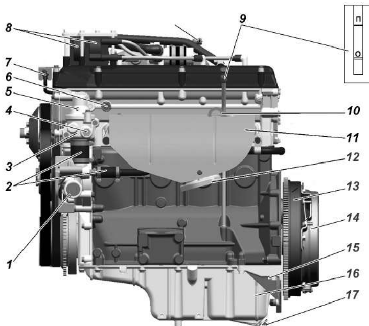
Рис. 9.10. Двигатель (вид слева):
