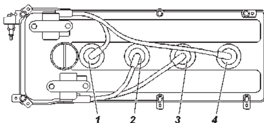
Рис. 9.14. Порядок установки высоковольтных проводов: 1, 2, 3, 4 -номера цилиндров двигателя
