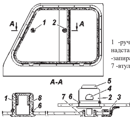
Рис. 3.7. Надставка двери:
