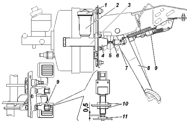
Рис. 9.17. Привод главного цилиндра выключения сцепления:
