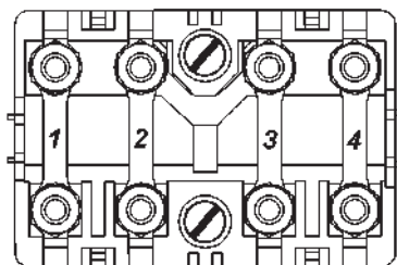
Рис. 9.41. Блок силовых плавких предохранителей:
