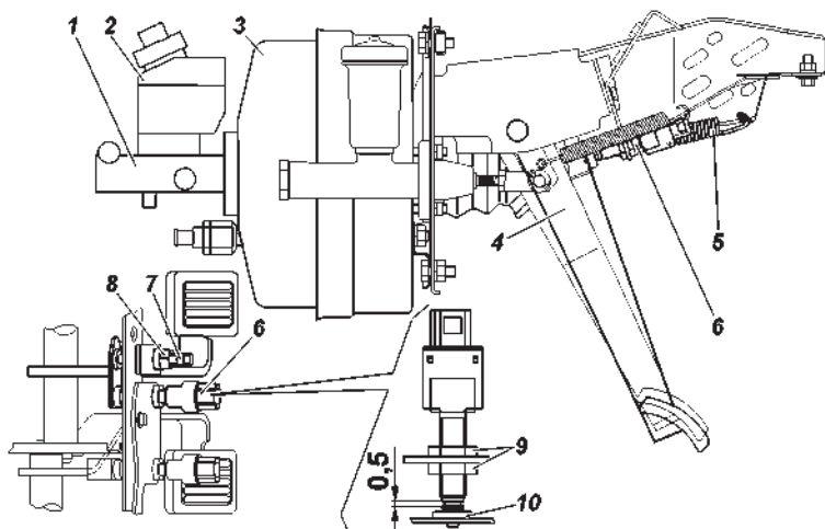
Рис. 9.34. Привод главного цилиндра:
