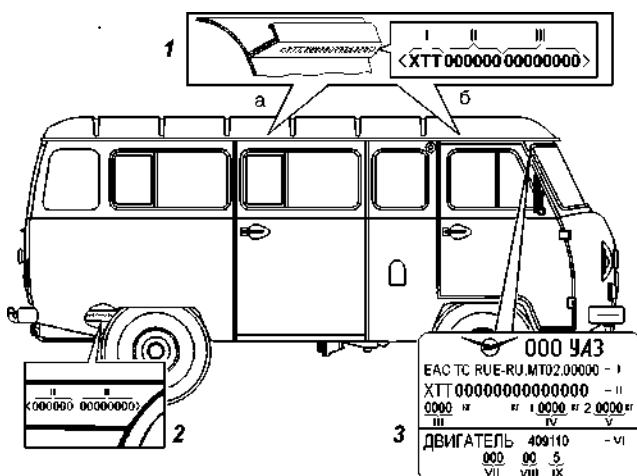
Рис. 1.12. Маркировка транспортного средства (ТС):
