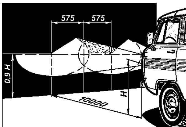
Рис. 9.39. Разметка экрана для регулировки фар:
