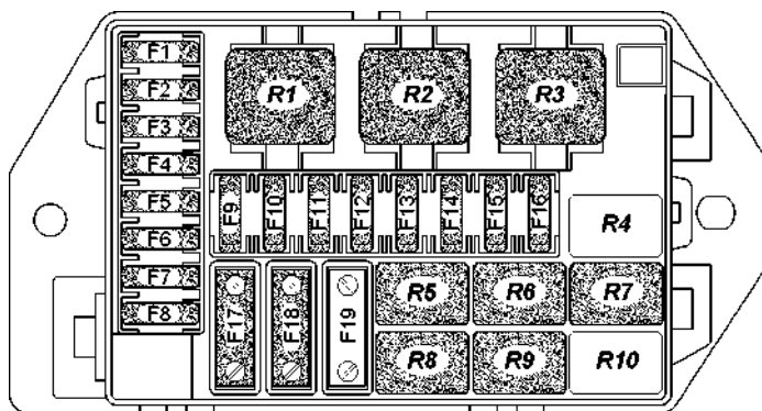
Рис. 9.36. Блок реле и предохранителей: R1-R10 -реле; F1-F19 -плавкие предохранители (см. таблицу 9.1)
