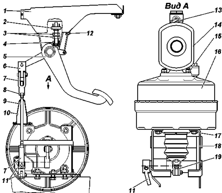
Рис. 9.32. Привод главного тормозного цилиндра:
