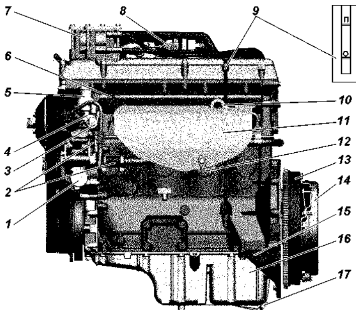
Рис. 9.2. Двигатель ЗМЗ-40911 (вид слева):
