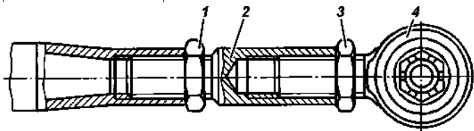
Рис. 9.23. Тяга рулевой трапеции:
