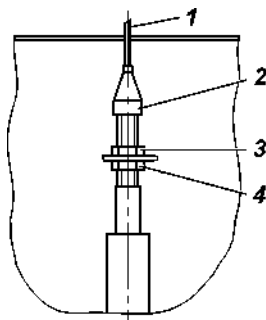
Рис. 9.8. Регулировка привода педали акселератора: 1 -трос; 2 -оболочка троса с регулировочным наконечником; 3, 4 -гайки
