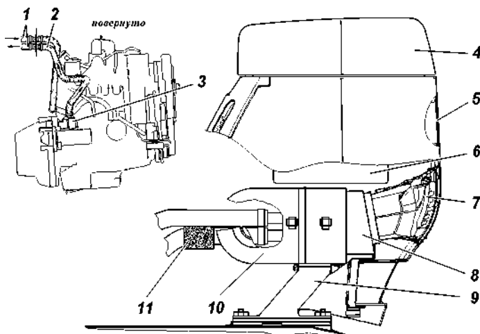
Рис. 3.35. Дополнительный отопитель:
