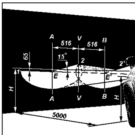
Рис. 9.34. Разметка экрана для регулировки фар: Н - расстояние центра фар от уровня земли; V-V - проекция продольной оси автомобиля; А-А, В-В - оси центров фар
