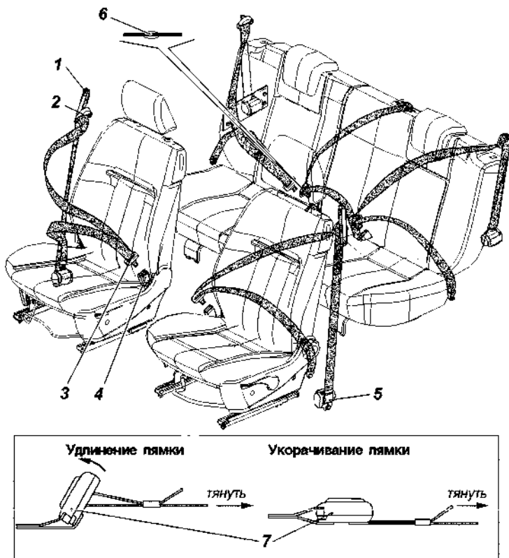
Рис. 3.48. Ремни безопасности:
