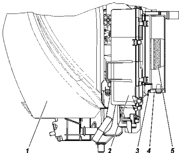
Рис. 3.37. Вентилятор:
