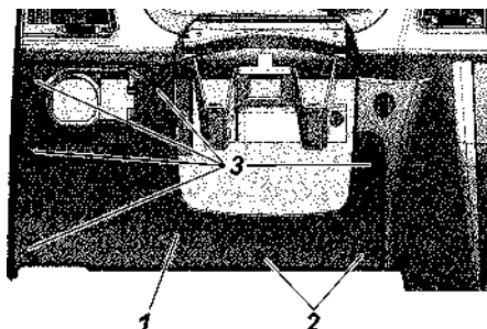
Рис. 9.31. Установка крышки блока реле и предохранителей : 1 -крышка блока реле и предохранителей; 2 -защелки крышки; 3 -клипсы крышки
