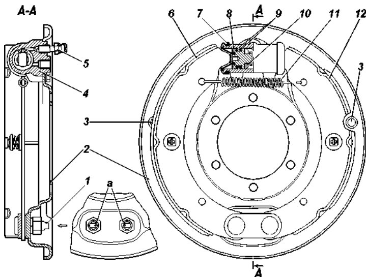
Рис. 9.26. Тормоз заднего колеса (Вариантное исп. 2): а -метки на опорных пальцах; 1 -опорные пальцы; 2 -щит; 3 -отверстия для визуального контроля состояния тормозных накладок; 4 -колесный тормозной цилиндр; 5 -перепускной клапан; 6,12 -тормозные колодки; 7 -защитный колпак; 8 -поршень; 9 -уплотнительные кольца; 10 -упорное кольцо; 11 -стяжная пружина
